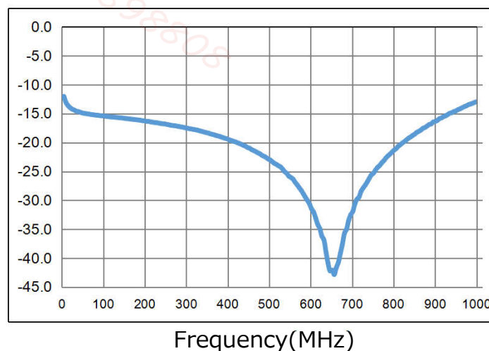
Input Return Loss(Pin1)
