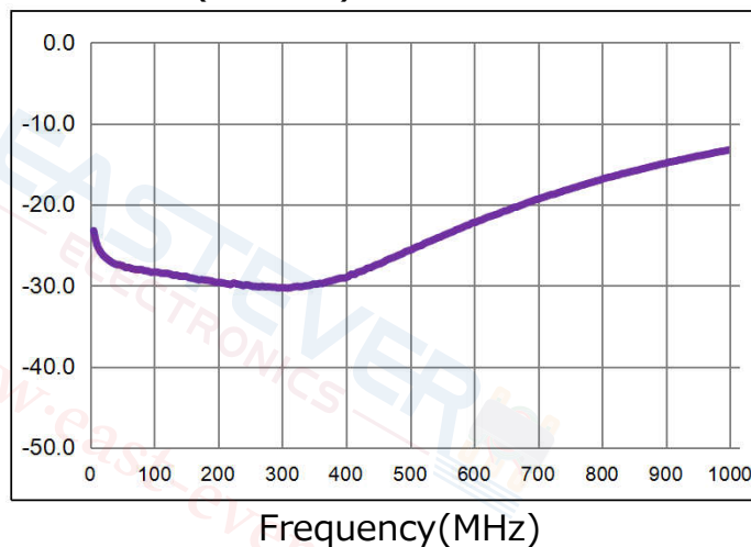
Isolation(Pin4-6)
