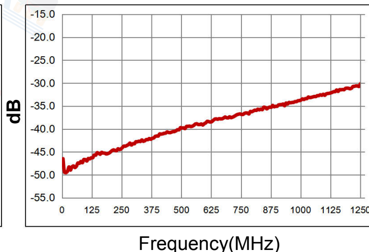
Isolation (Pin1-4)
