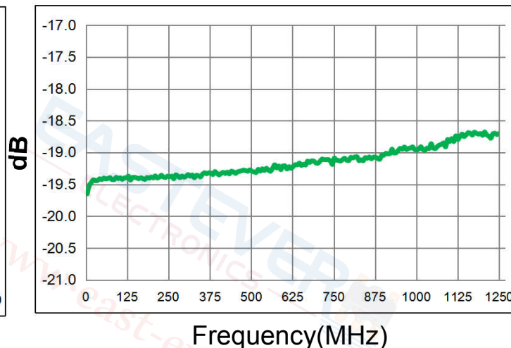
Coupling(pin1-3):
